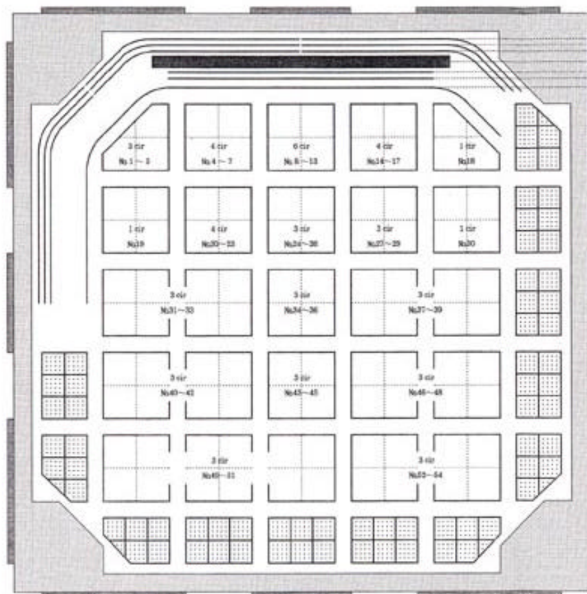
フライフレーム配置図
